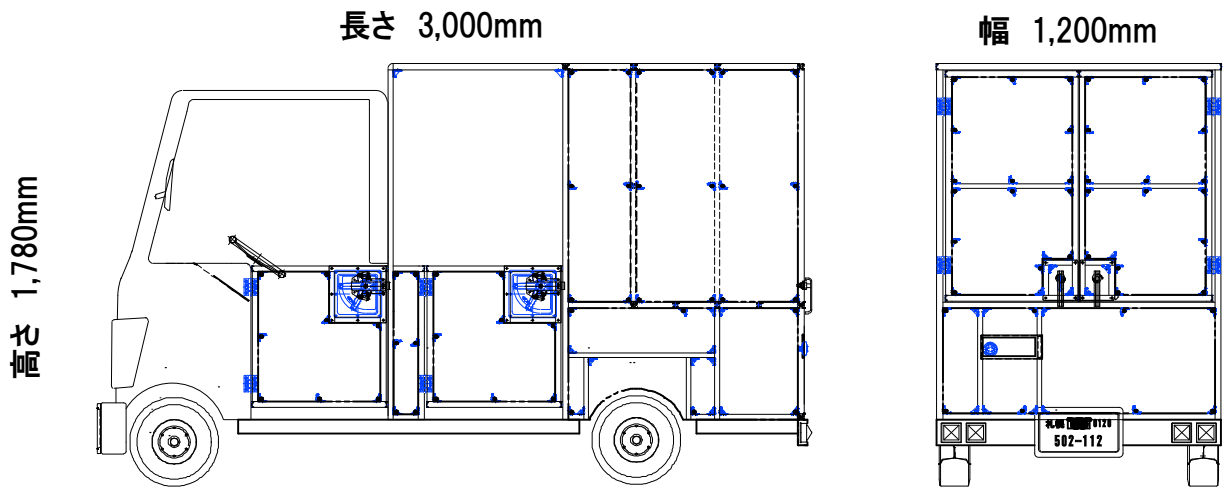
車両寸法図
